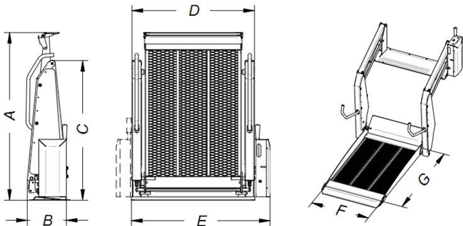
Габаритные размеры
