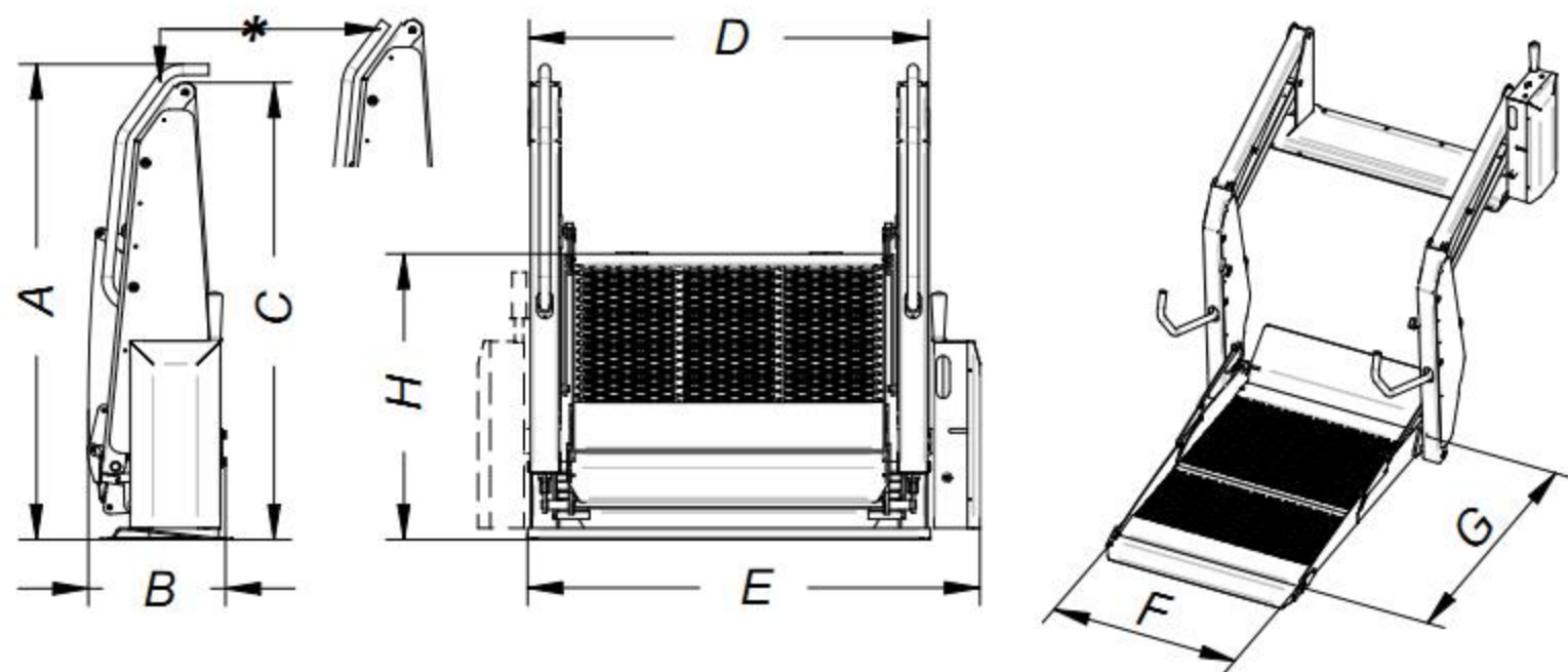
Габаритные размеры
