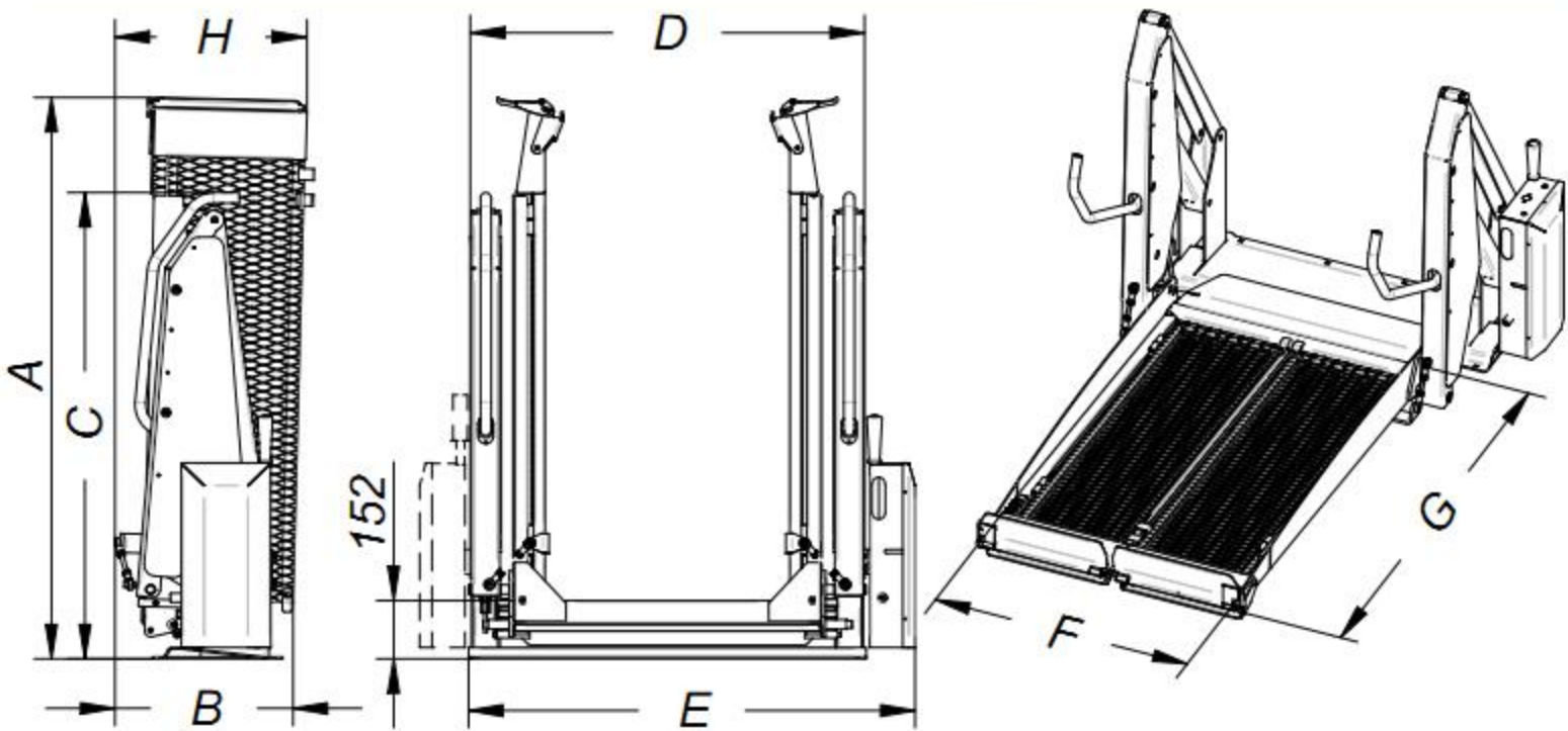
Габаритные размеры
